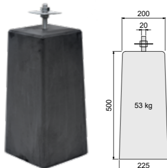
Betonpoer XL
